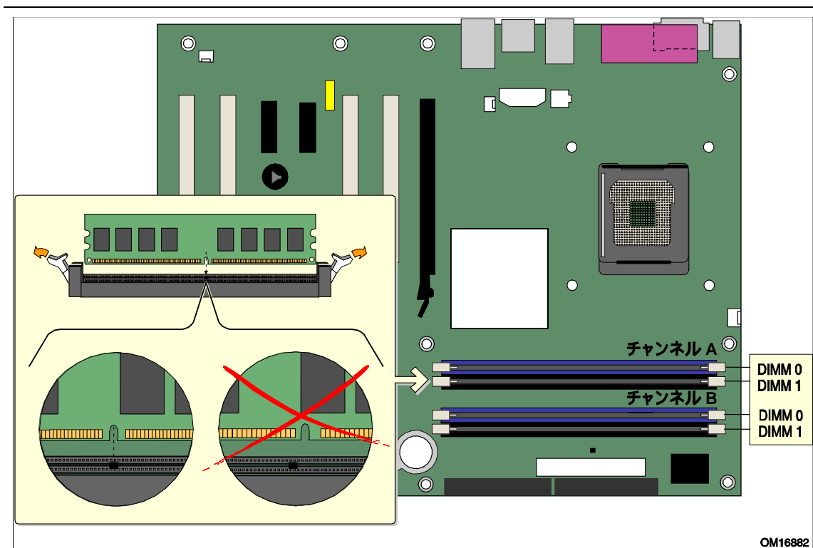
図 17. DIMM の取り付け
