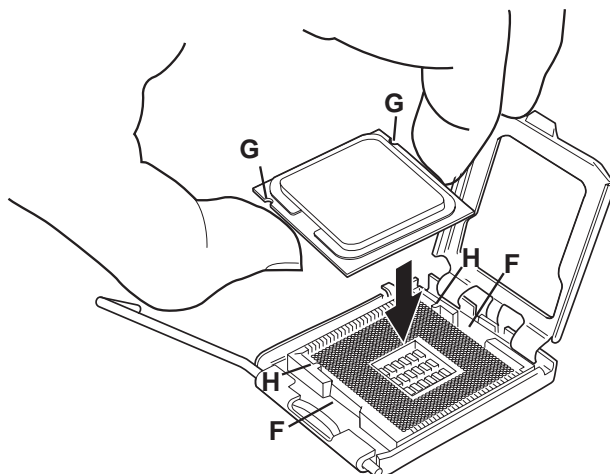
図 10. プロセッサの取り付け
