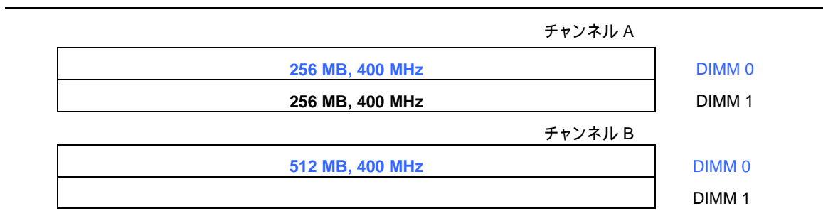
図 15. デュアル構成の例 3
