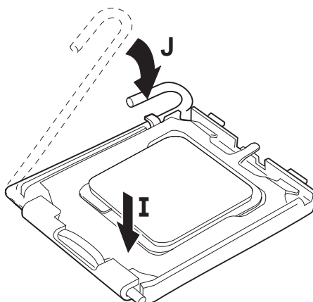
図 11. ロード・プレートを閉じる
