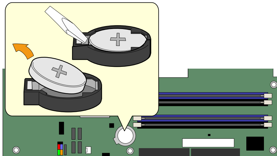
図 29. 電池の取り外し
