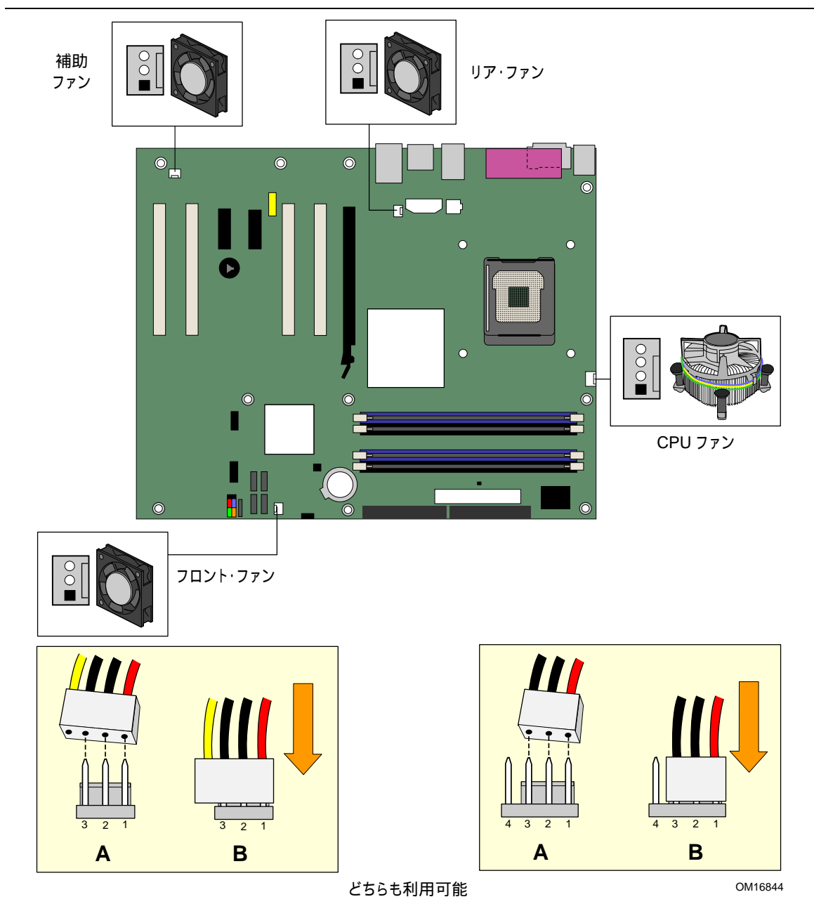
図 23. ファン・ヘッドの位置
