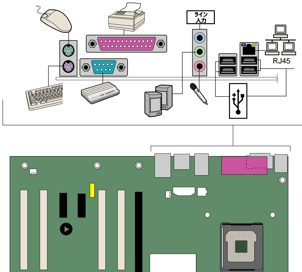
図 28. バック・パネル・コネクタ
