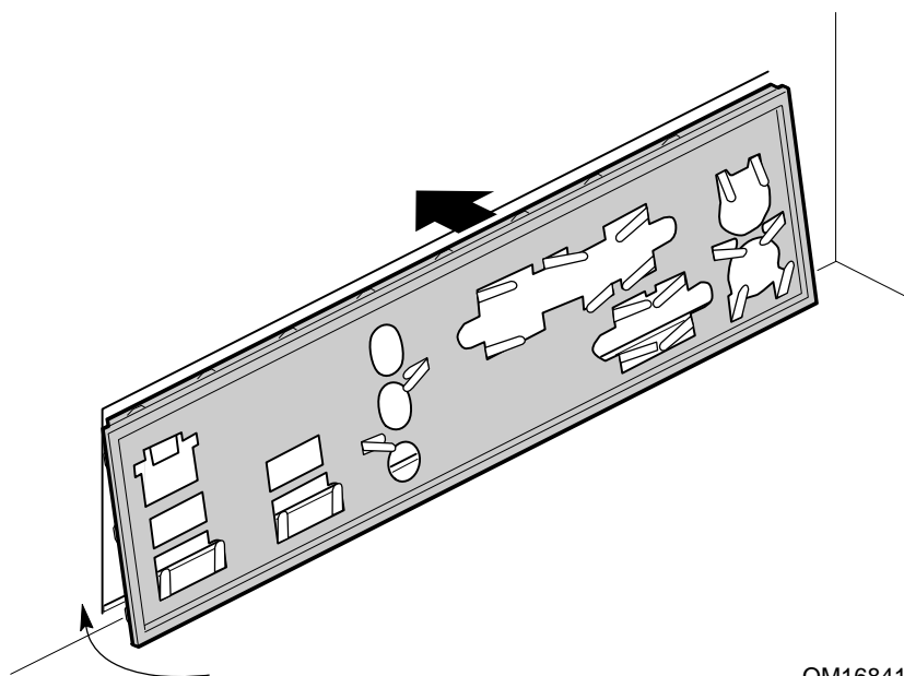
図 4. I/O シールドの取り付け
