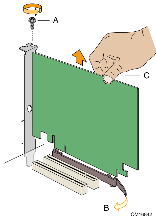
図 18. PCI Express x16 カードの取り外し
