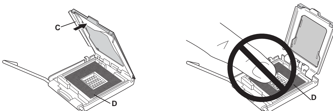
図 7. ロード・プレートを持ち上げる(ソケットの接点には触れないこと)
