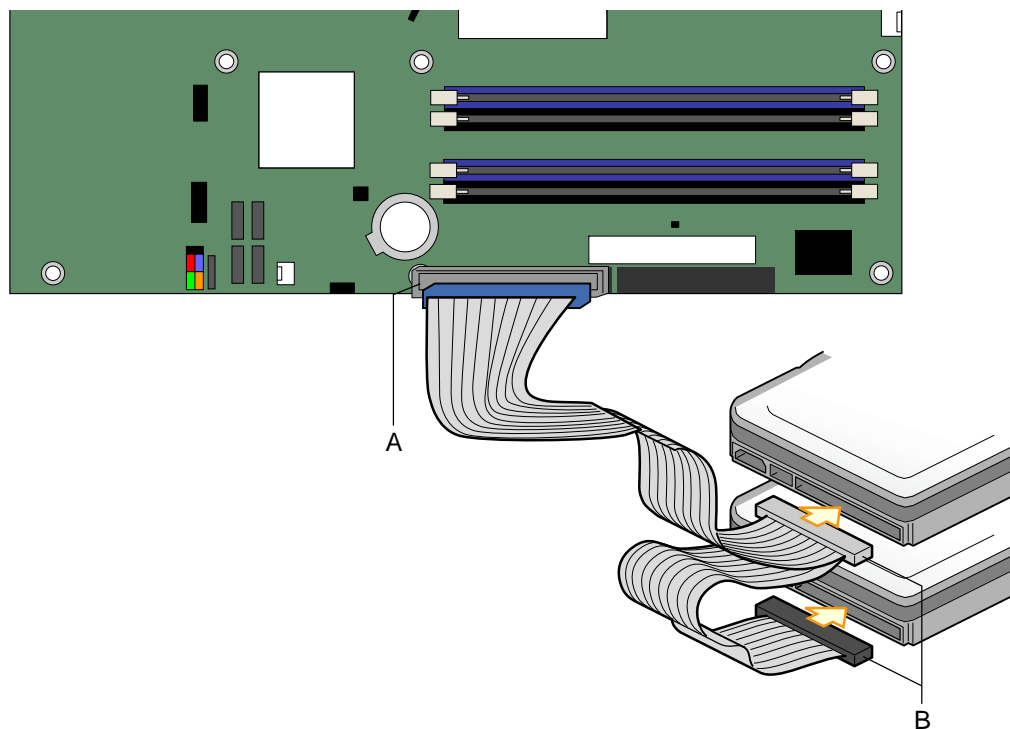
図 19. IDE ケーブルの接続
