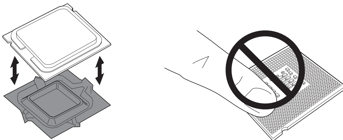
図 9. プロセッサを保護カバーから取り外す
