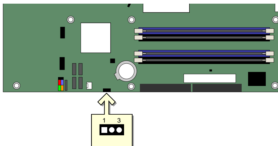
図 27. BIOS コンフィギュレーション・ジャンパ・ブロックの位置
