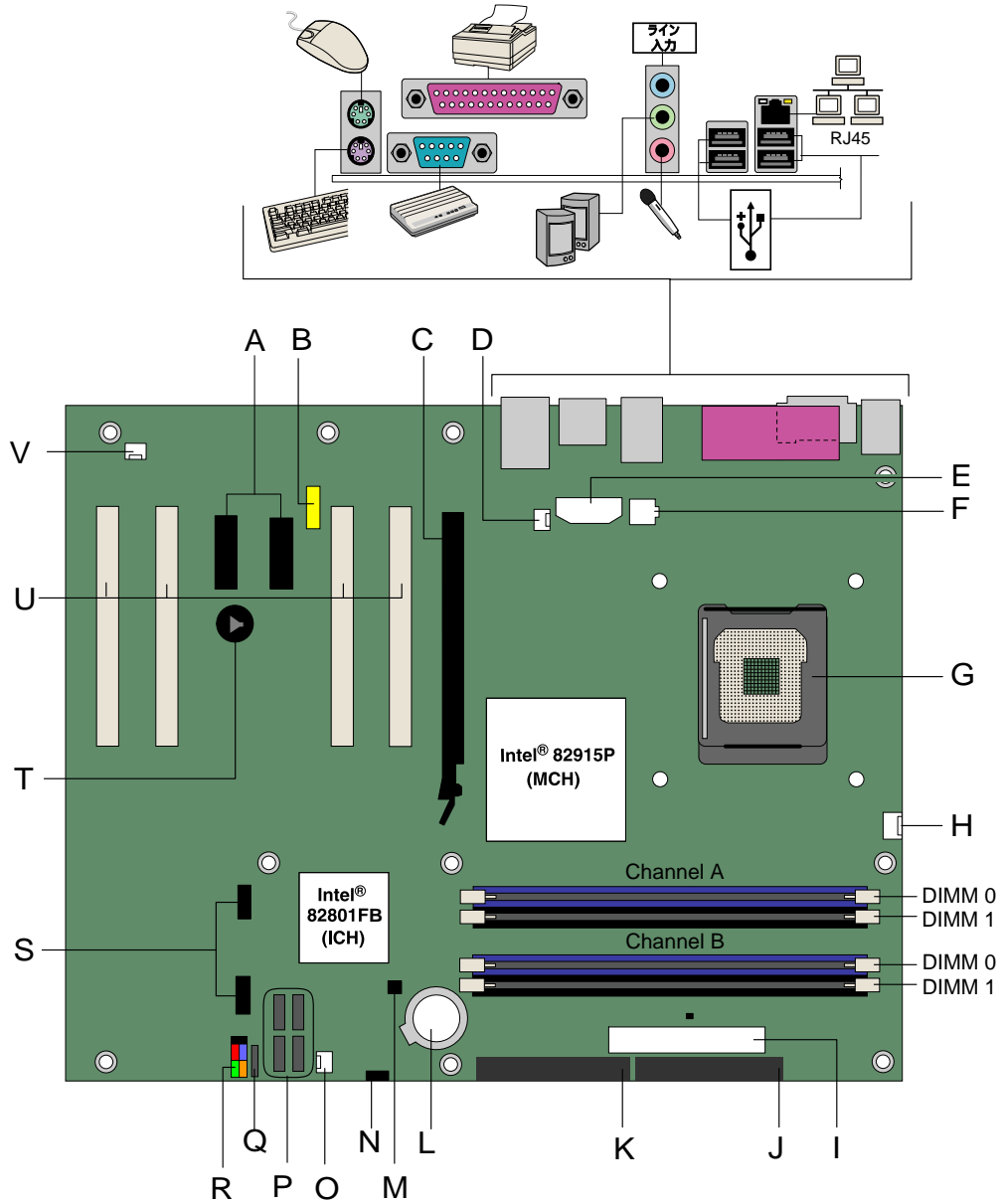
図 1. デスクトップ・ボード D915PGN および D915PCY のコンポーネント
