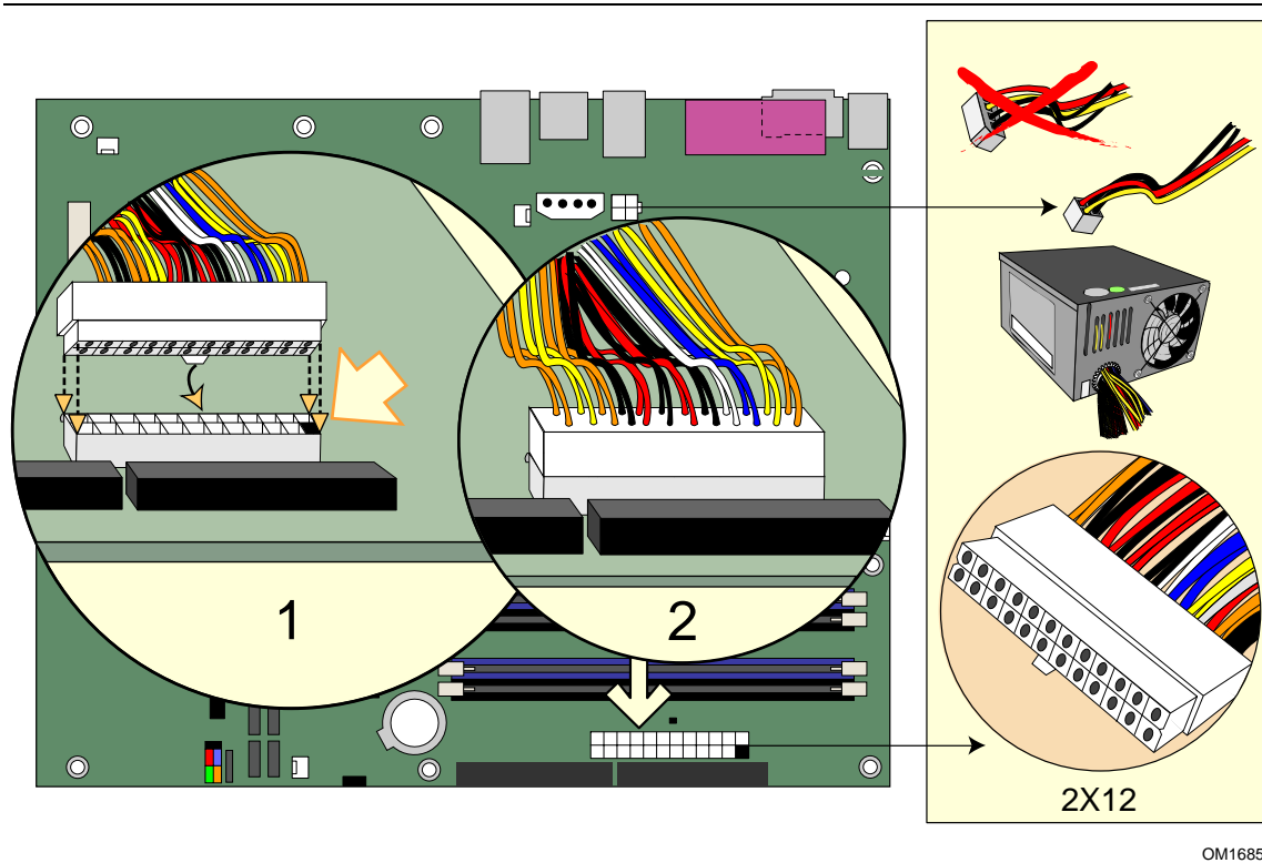
図 25. 2x12 電源ケーブルの接続
