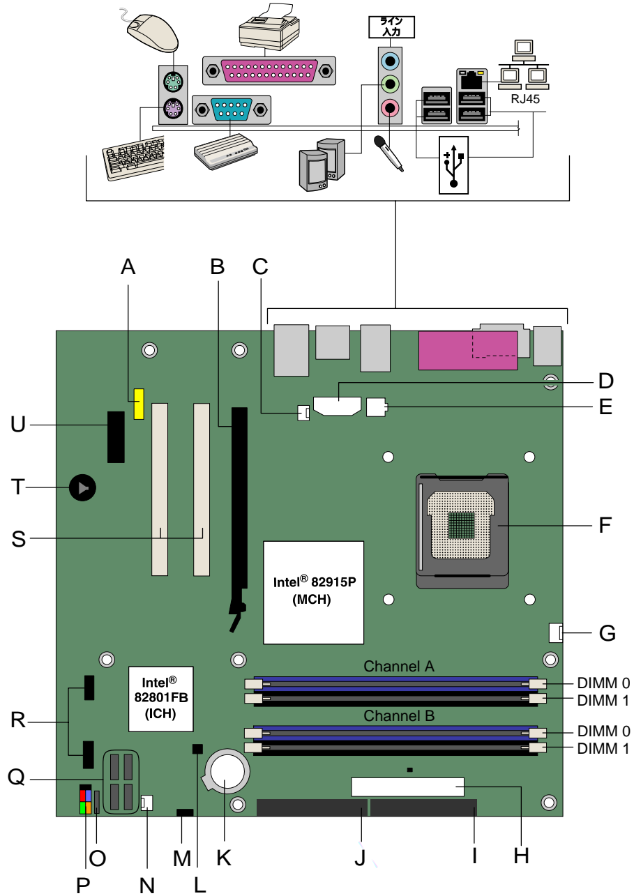
図 2. インテル・デスクトップ・ボード D915PSY および D915PCM のコンポーネント
