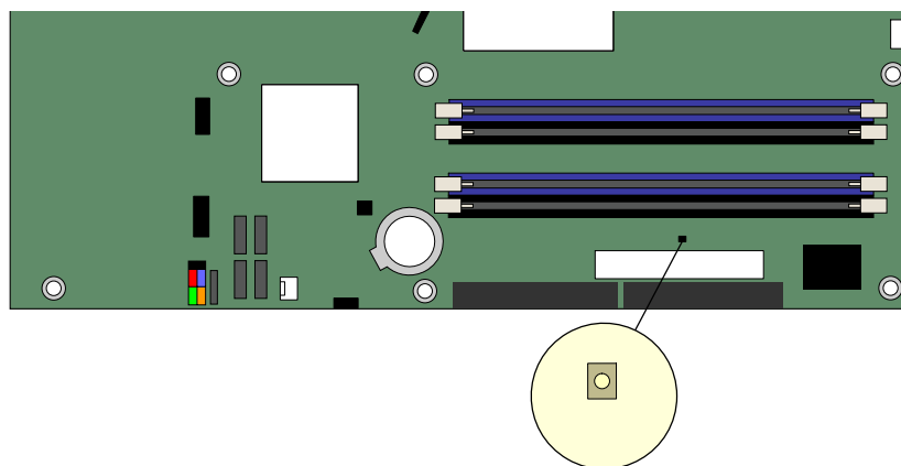
図 3. スタンバイ電源インジケータの位置
