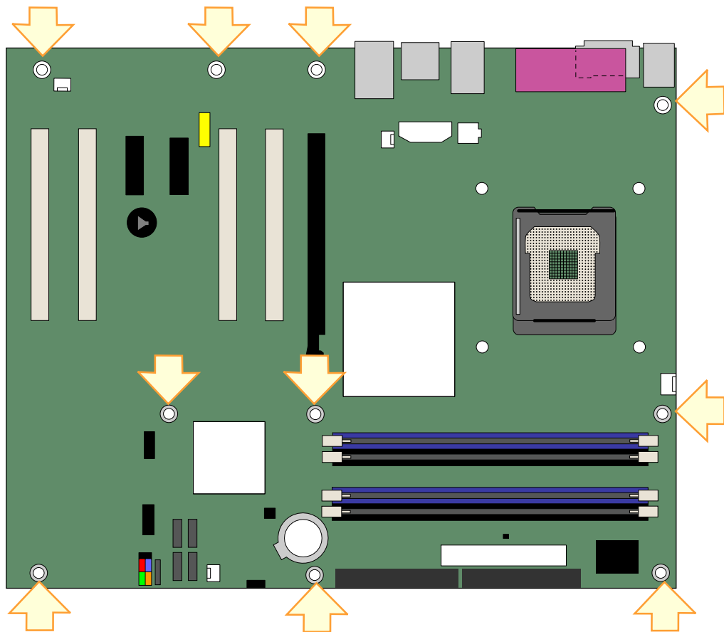
図 5. デスクトップ・ボード D915PGN および D915PCY の取り付けネジ穴の位置
