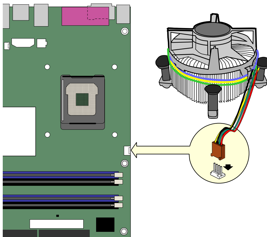
図 12. プロセッサ・ファン・ヒートシンク・ケーブルをプロセッサ・ファン・コネクタに接続
