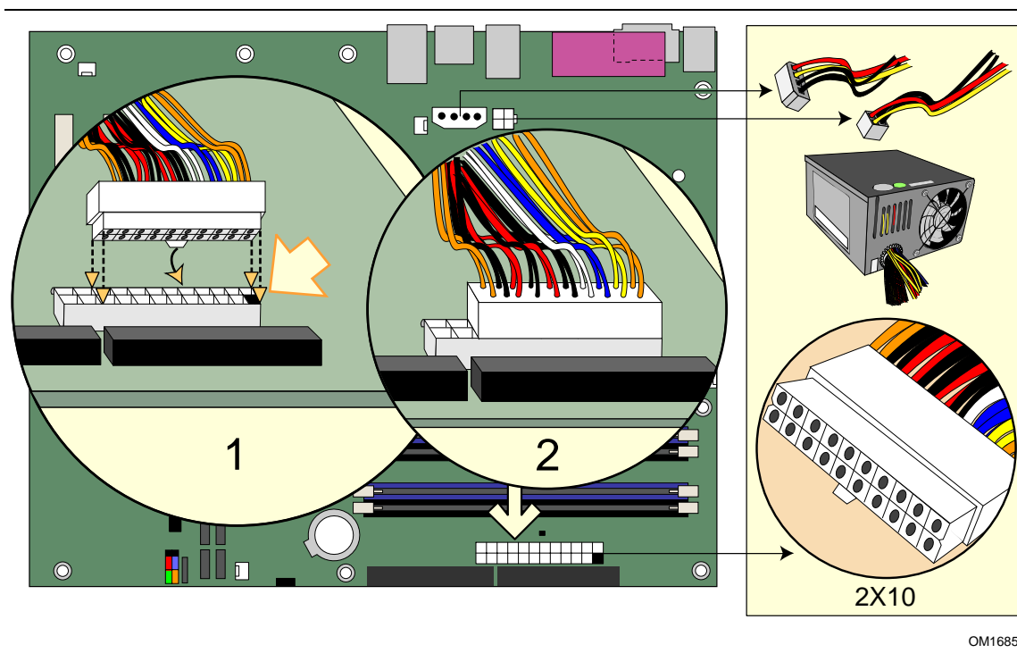
図 24. 2x10 電源ケーブルの接続
