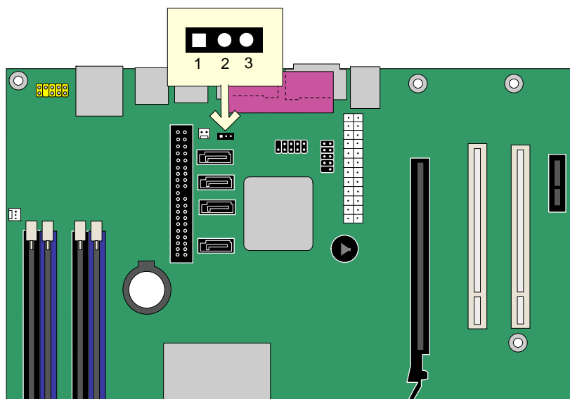
図 25. BIOS コンフィグレーション・ジャンパの位置
