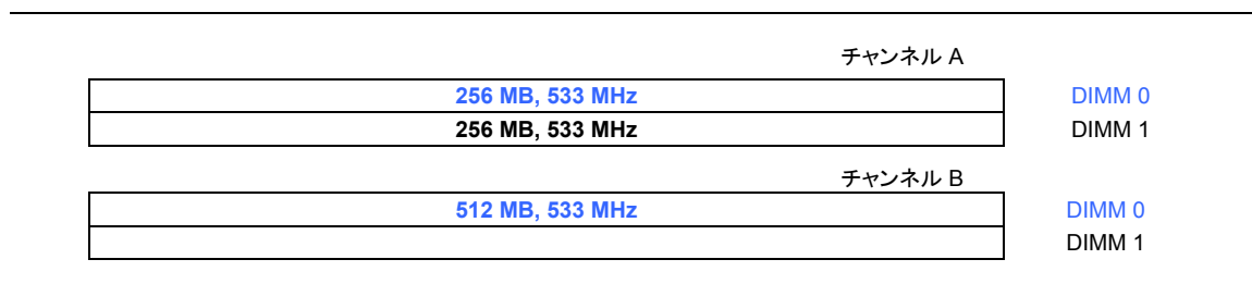
図 15. デュアルチャンネル・メモリ構成の例 3
