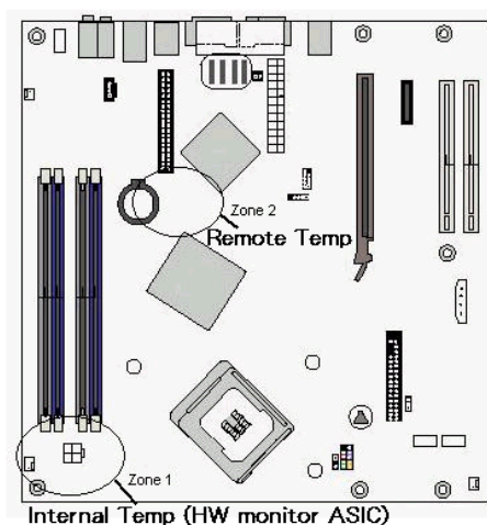
温度センサーの配置図
