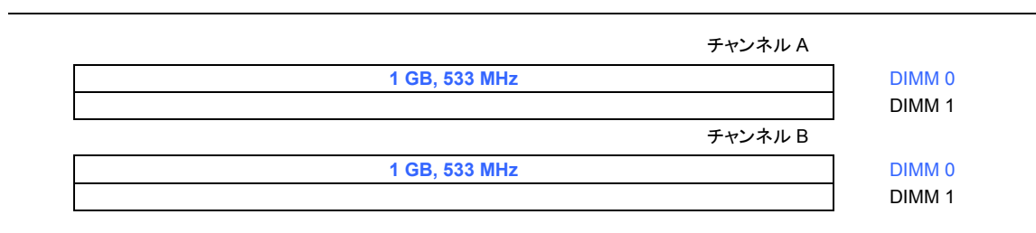
図 13. デュアルチャンネル・メモリ構成の例 1
