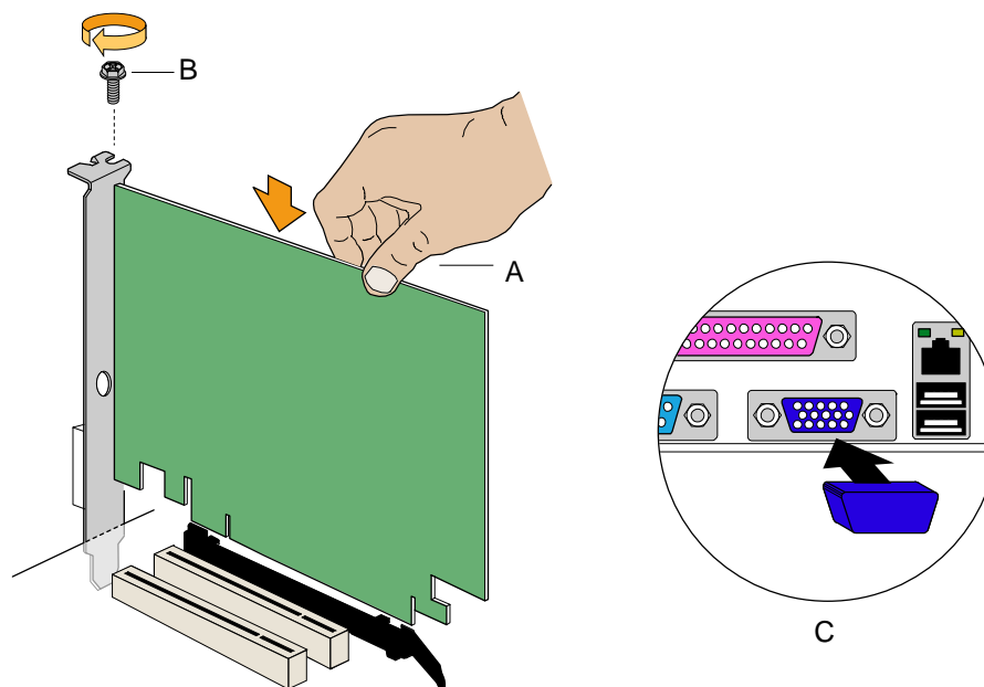
図 17. PCI Express x16 カードを挿入し、リア・パネル VGA ポートにカバーを装着
