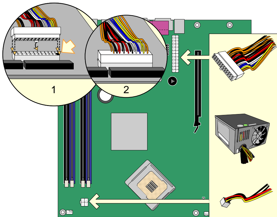
図 23. 電源ケーブルの接続
