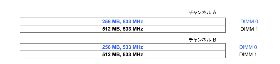
図 14. デュアルチャンネル・メモリ構成の例 2
