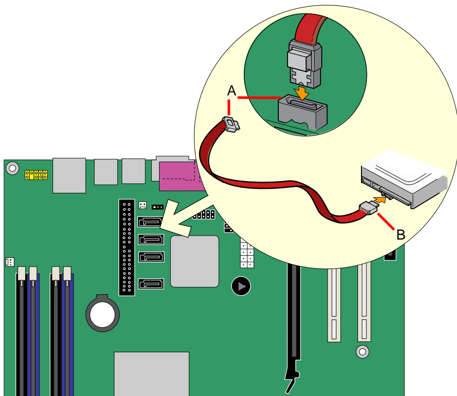
図 19. シリアル ATA ケーブルの接続
