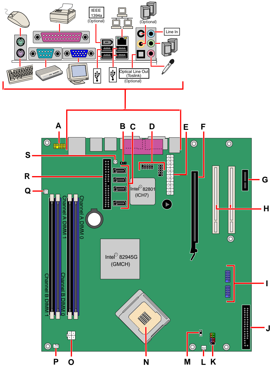
図 1. デスクトップ・ボード D945GCZ のコンポーネント
