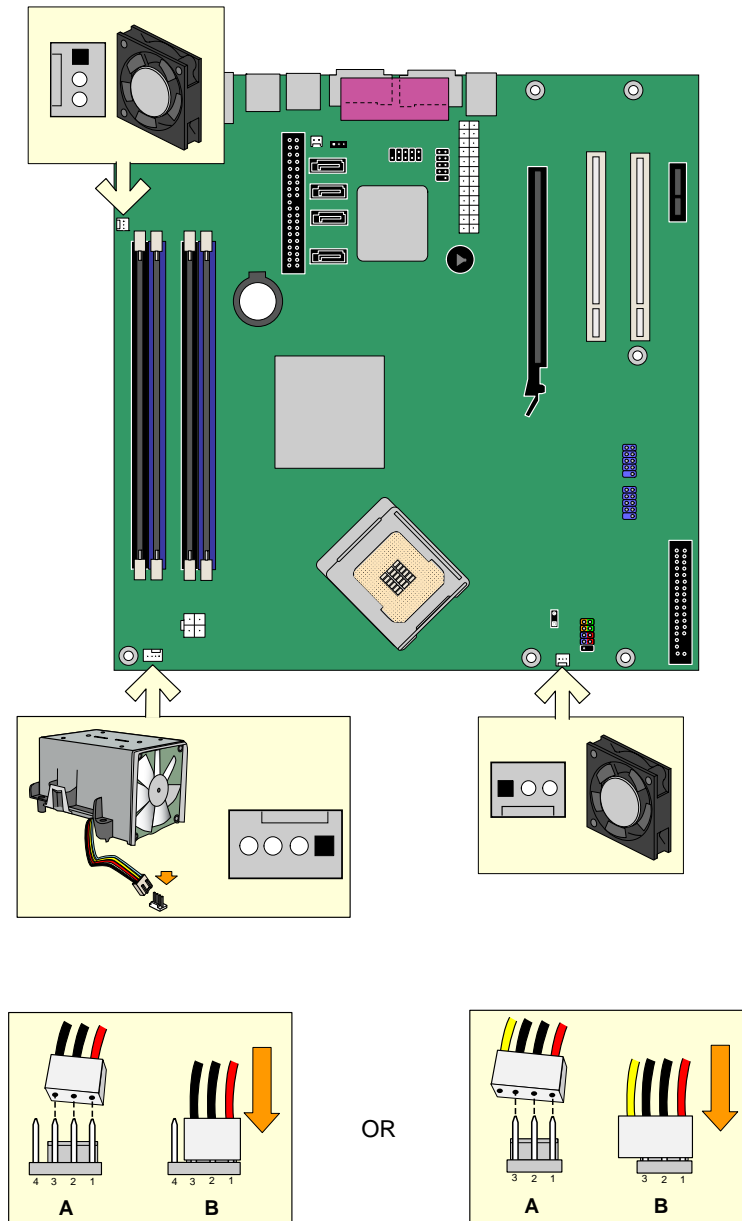
図 22. ファン・ヘッドの位置 (ピン数の合わないケーブルの接続例)
