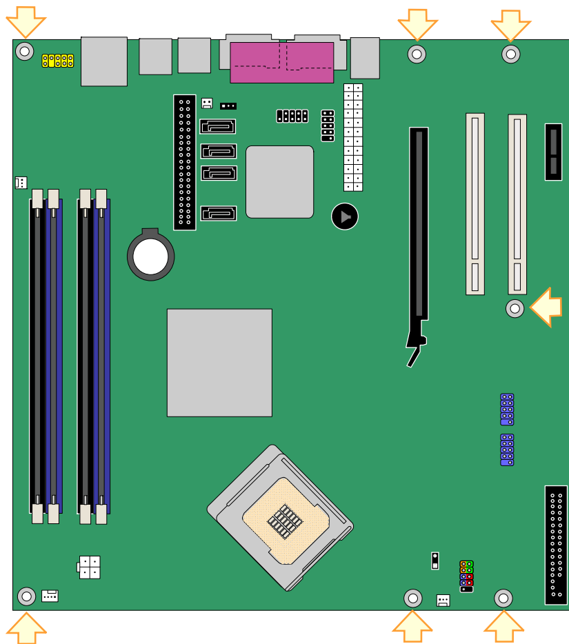
図 5. デスクトップ・ボード D945GCZ の取り付けネジ穴の位置
