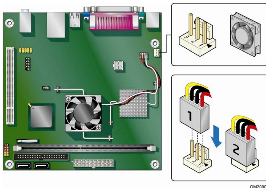
图 12. 机箱风扇接头连接器位置
