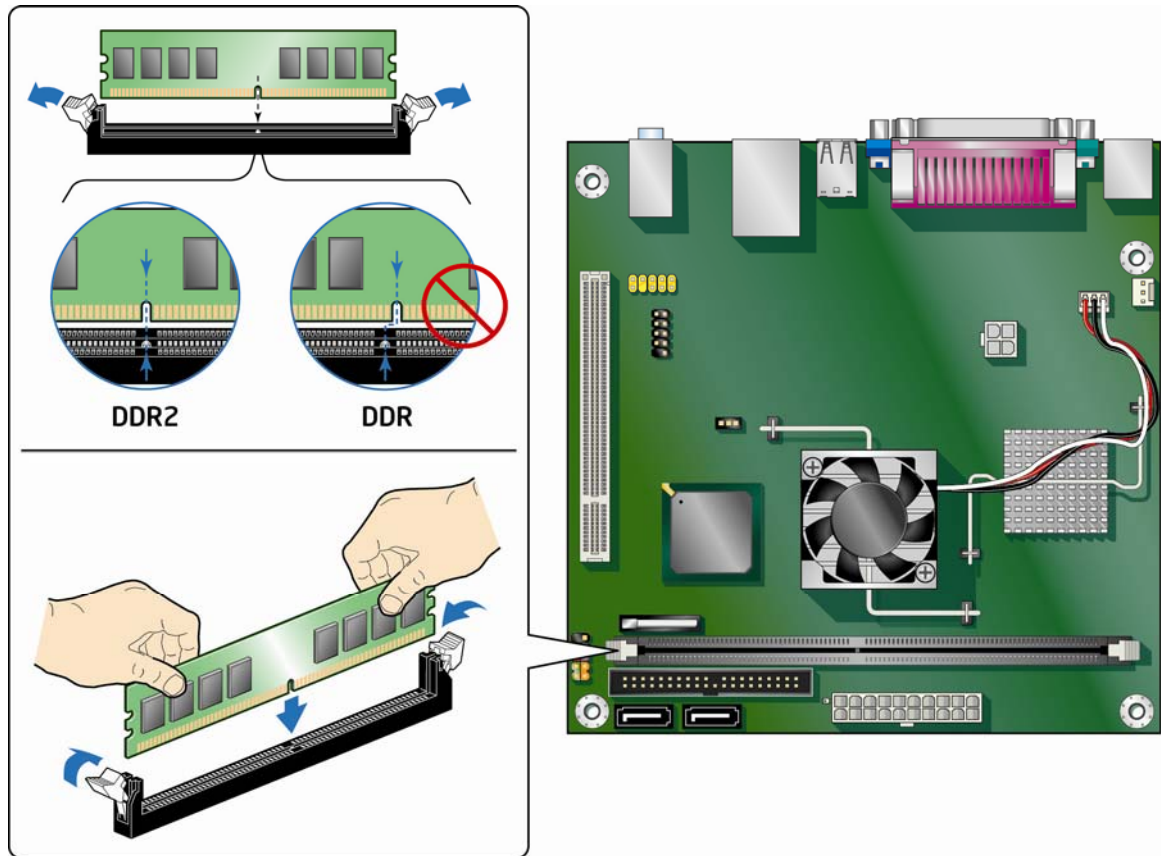
图 8. 安装 DIMM
