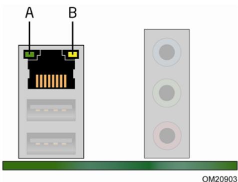
图 3. LAN 状态 LED 指示灯
