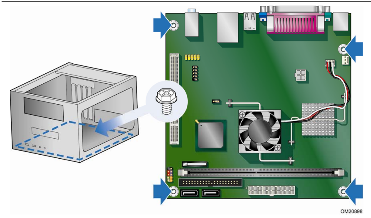
图 6. 台式机主板 DG945GCLF 安装螺丝孔
