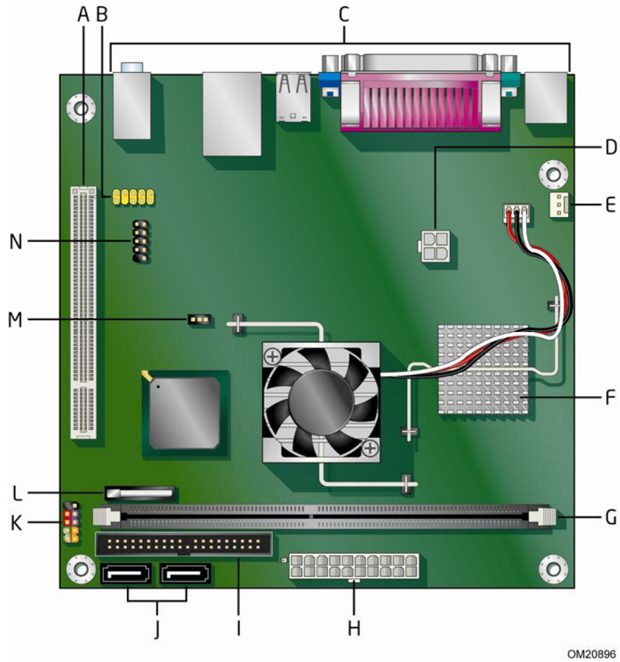
图 1. 英特尔台式机主板 DG945GCLF 组件
