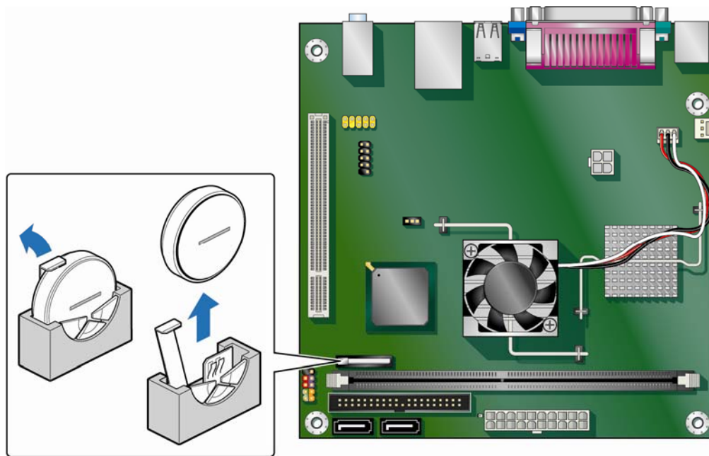
图 15. 拆卸电池
