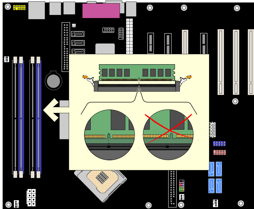
图 17. 安装 DIMM
