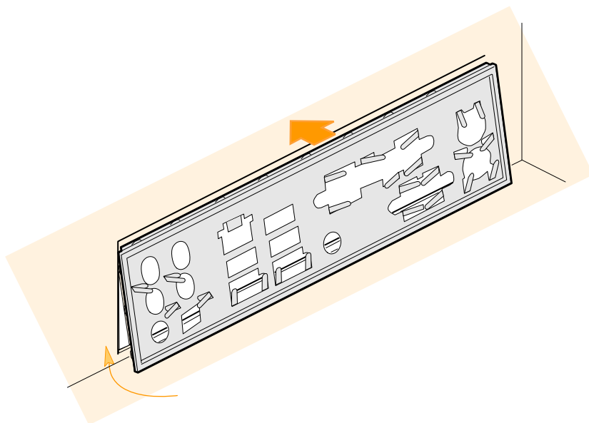
图 4. 安装 I/O 防护板
