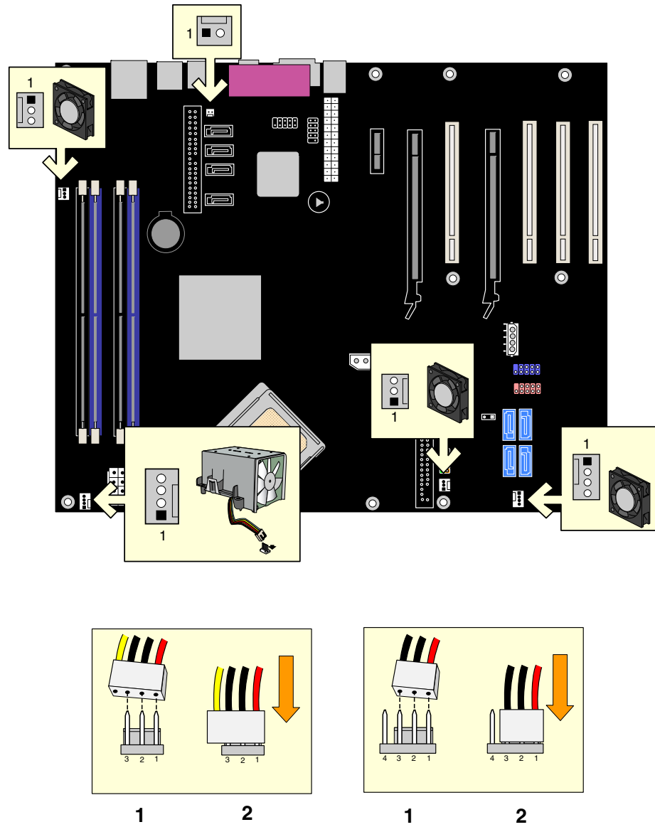
图 25. 风扇和机箱开启接头连接器位置
