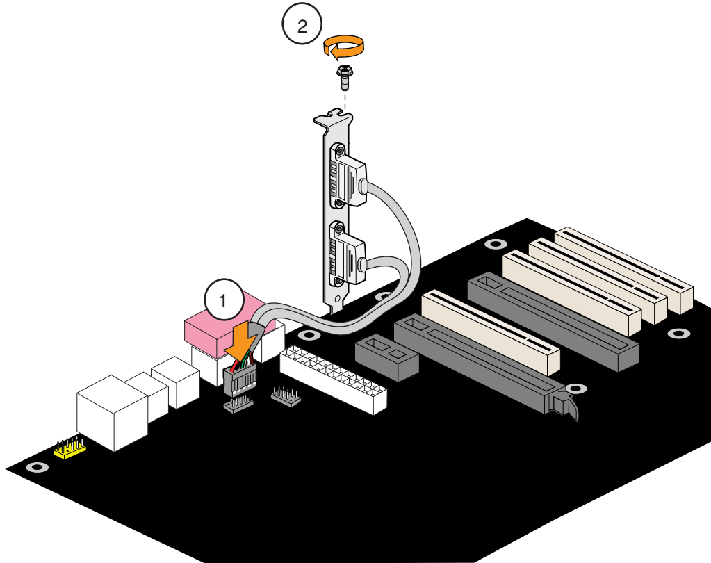
图 23. 连接背面板高速 USB 2.0 适配器
