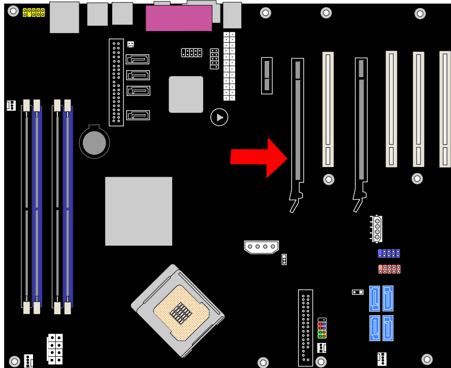
图 18. 用于一块视频卡的槽
