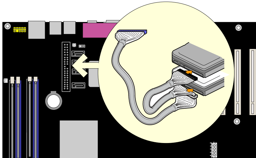
图 20. 连接 IDE 电缆
