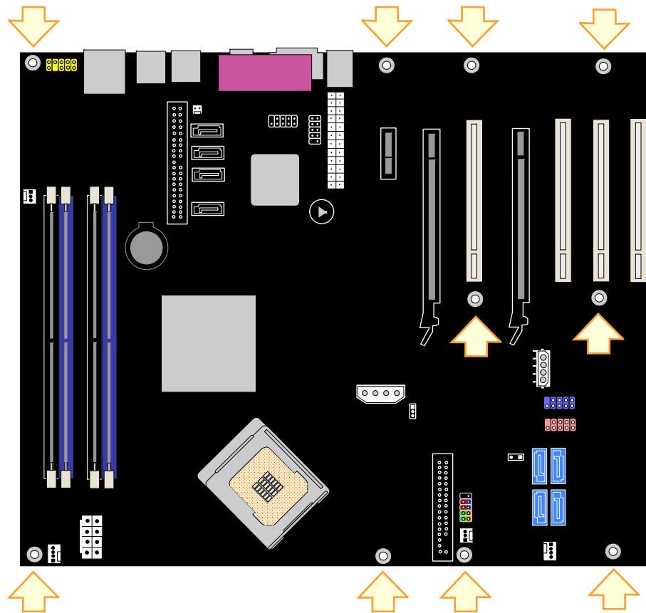
图 5. 安装螺丝孔位置
