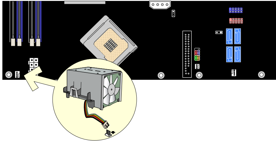
图 12. 将处理器风扇散热器电缆连接到处理器风扇接头连接器上
