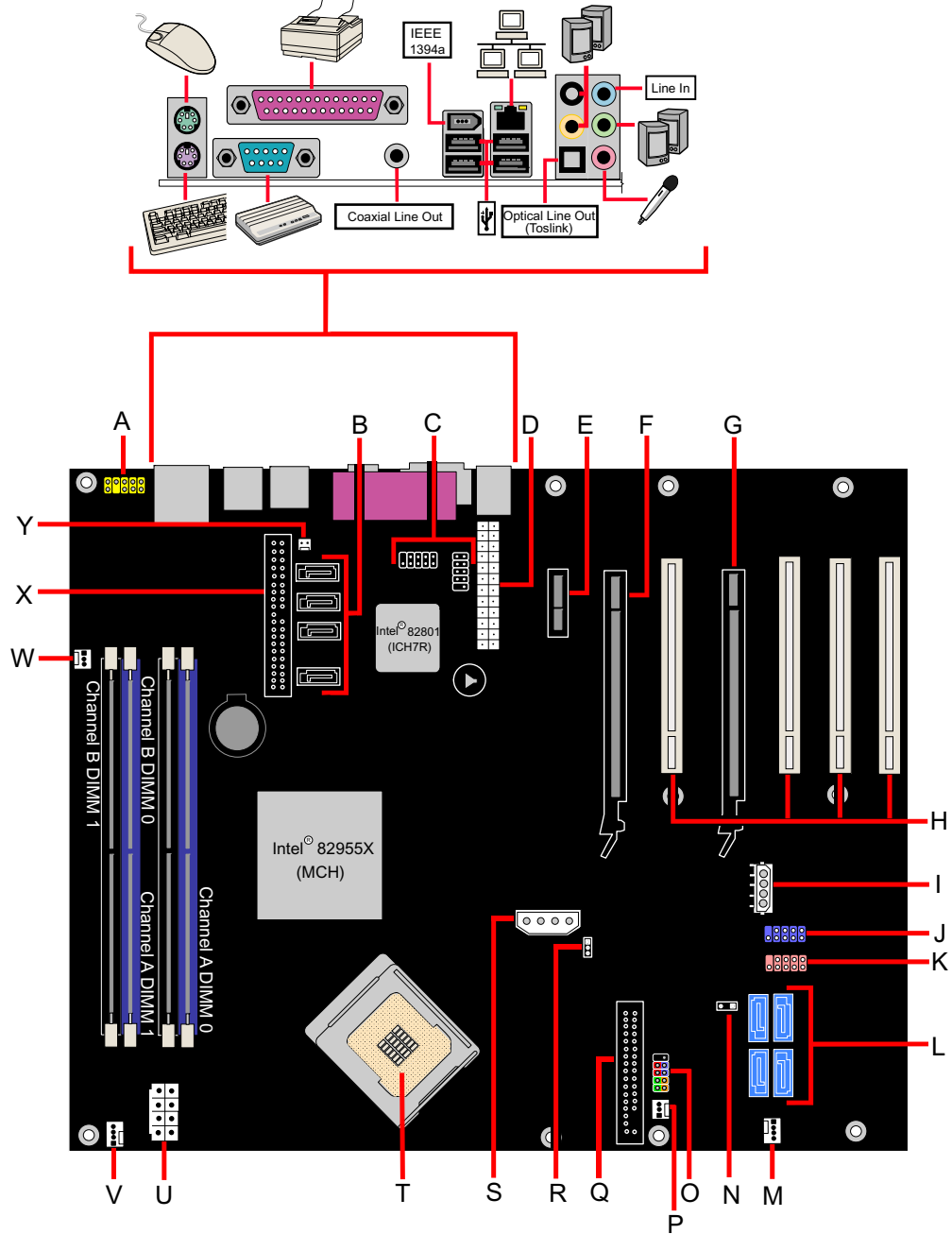
图 1. 台式机主板 D955XCS 组件
