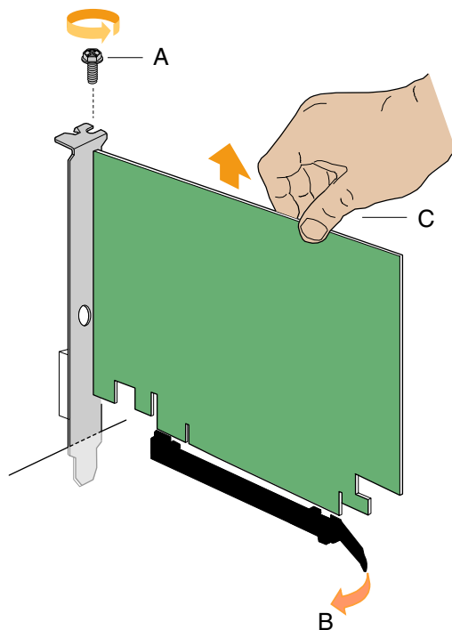
图 19. 拆卸 PCI Express x16 卡
