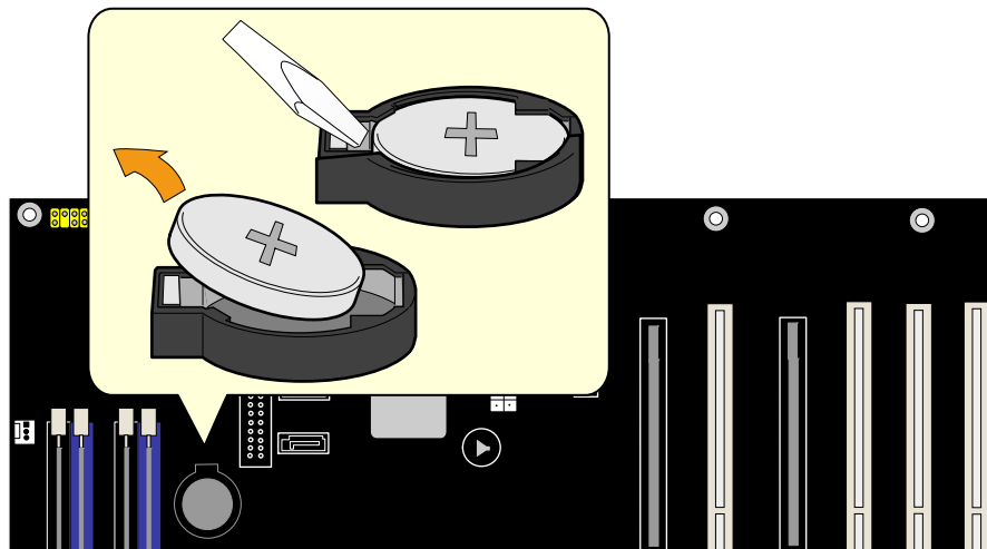
图 32. 拆卸电池
