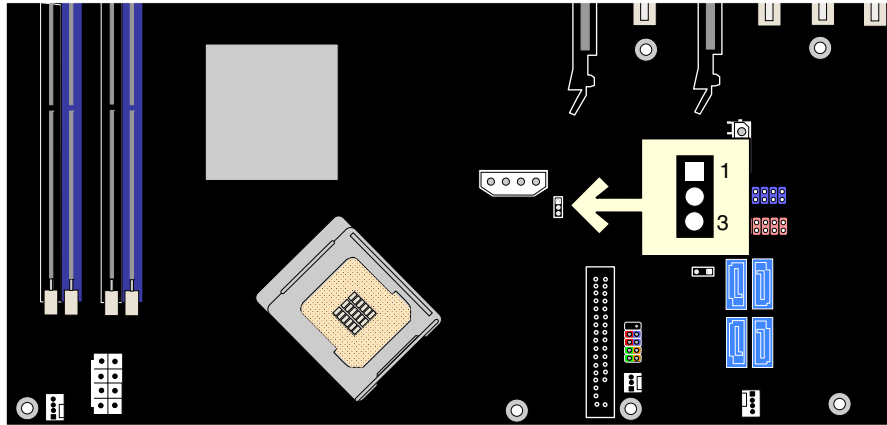
图 30. BIOS 配置跳线块位置
